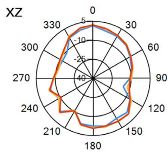
— 2.4GHz — 2.45GHz — 2.5GHz
